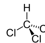
Chloroform CHCl 3
