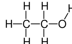
Ethanol C 2 H 6 O
